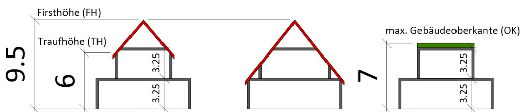
Abb. 14 Abb.: Schema der festgesetzten maximalen Gebäudehöhen
